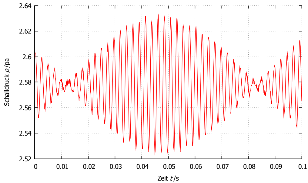
Abbildung 2: Schwebung mit f_1 = 440\text{Hz} und f_2 = 410\text{Hz}
